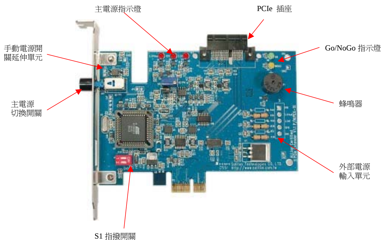
PEX-1X 電路板圖示
